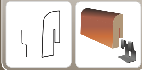
Lišta soklová 40 x 14 mm + klip Omán
