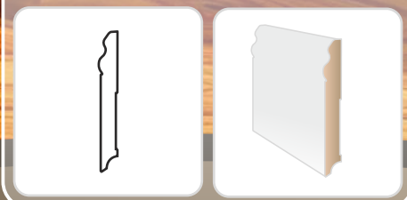
KP 120 120 x 14 mm
