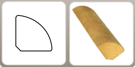
Čtvrtekroužek - PO5 15 x 15 mm
